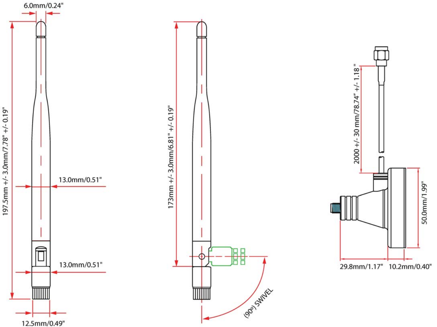
ANT18769 天线、底座和电缆尺寸
